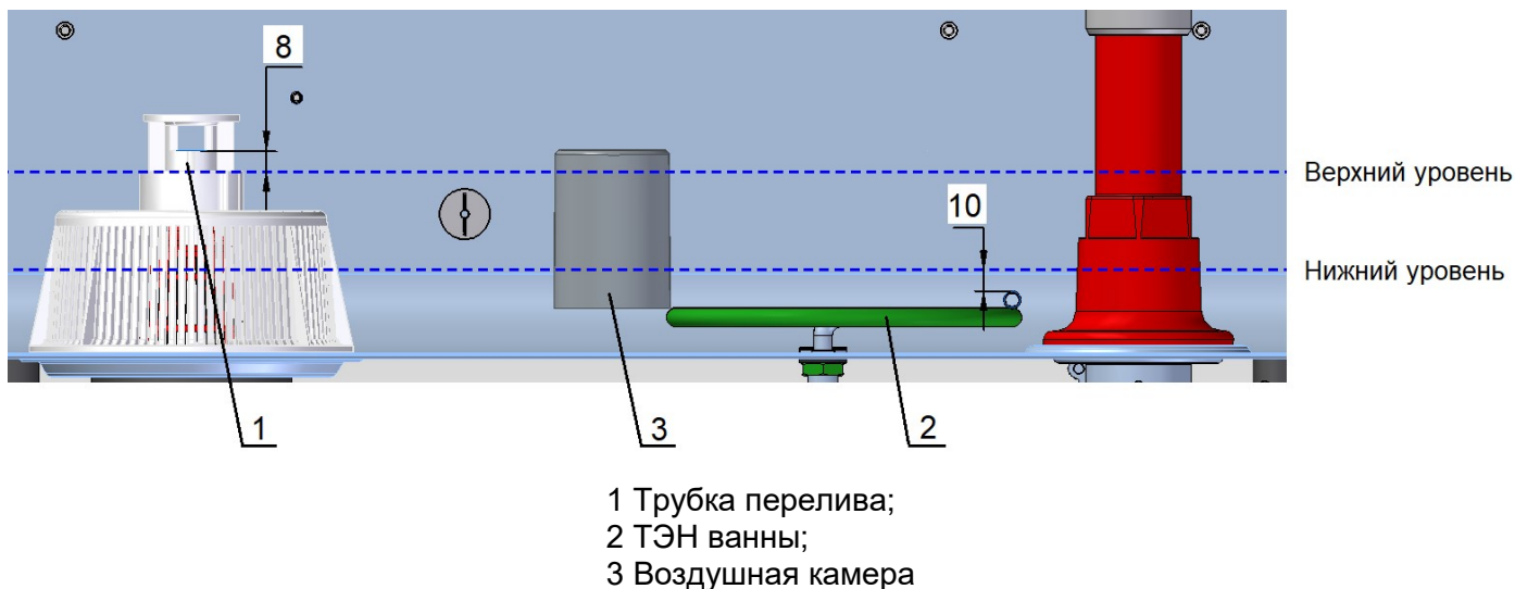
Рис. 4 «Верхний» и «нижний» уровни воды в ванне
