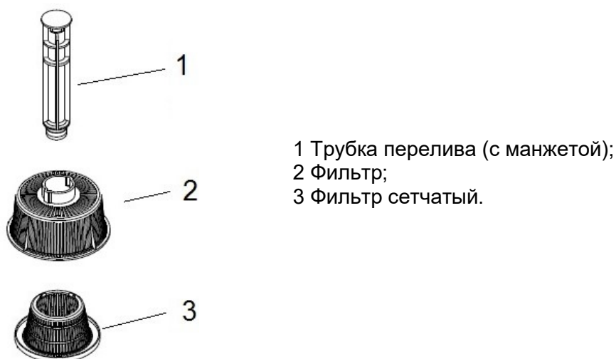
Рис. 2 Трубка перелива с фильтрами
