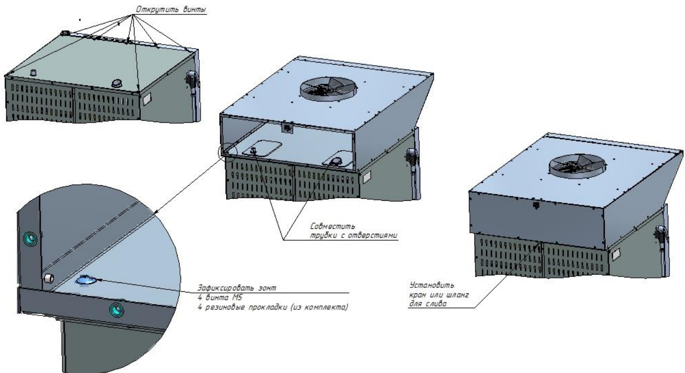
Рис.3 Установка зонта на пароконвектомат
