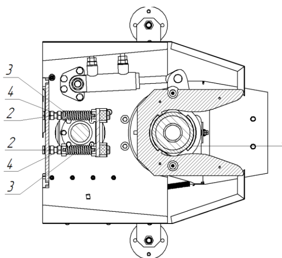
Рис.7 Регулировка механизма захвата дежи.
