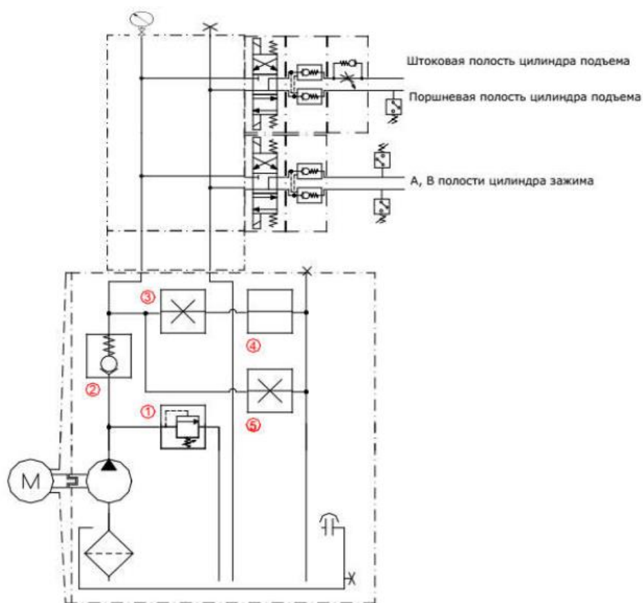
Рис.9 Гидравлическая схема машины.
