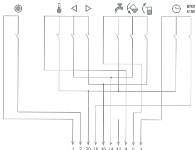
Рис. 8 Схема пленочной клавиатуры
