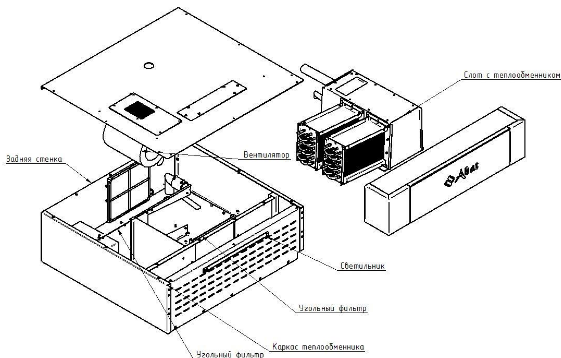
Рис 3 - Состав зонта
