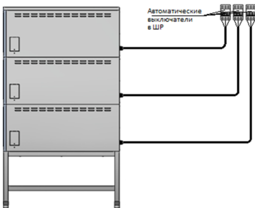
Рис.5 Схема подключения ЭШП-3-01КП 3EN Super с парогенератором к сети
