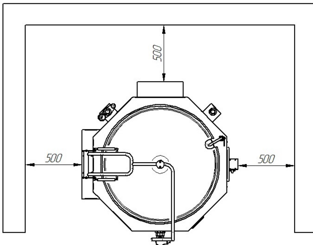
Рисунок 2 Установка котла
