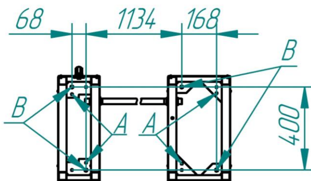
Рис. 5 Размеры для сверления крепежных болтов к полу
