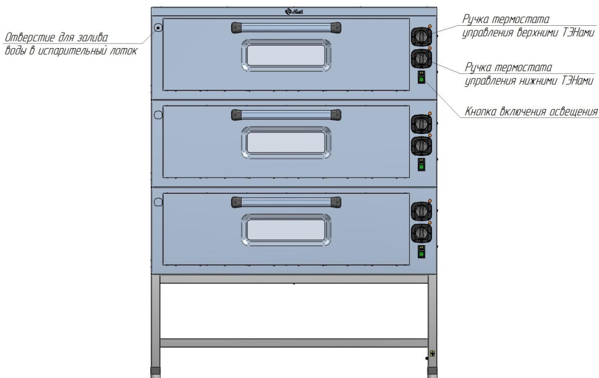
Рис. 4. Органы управления ЭСП-3-01.
